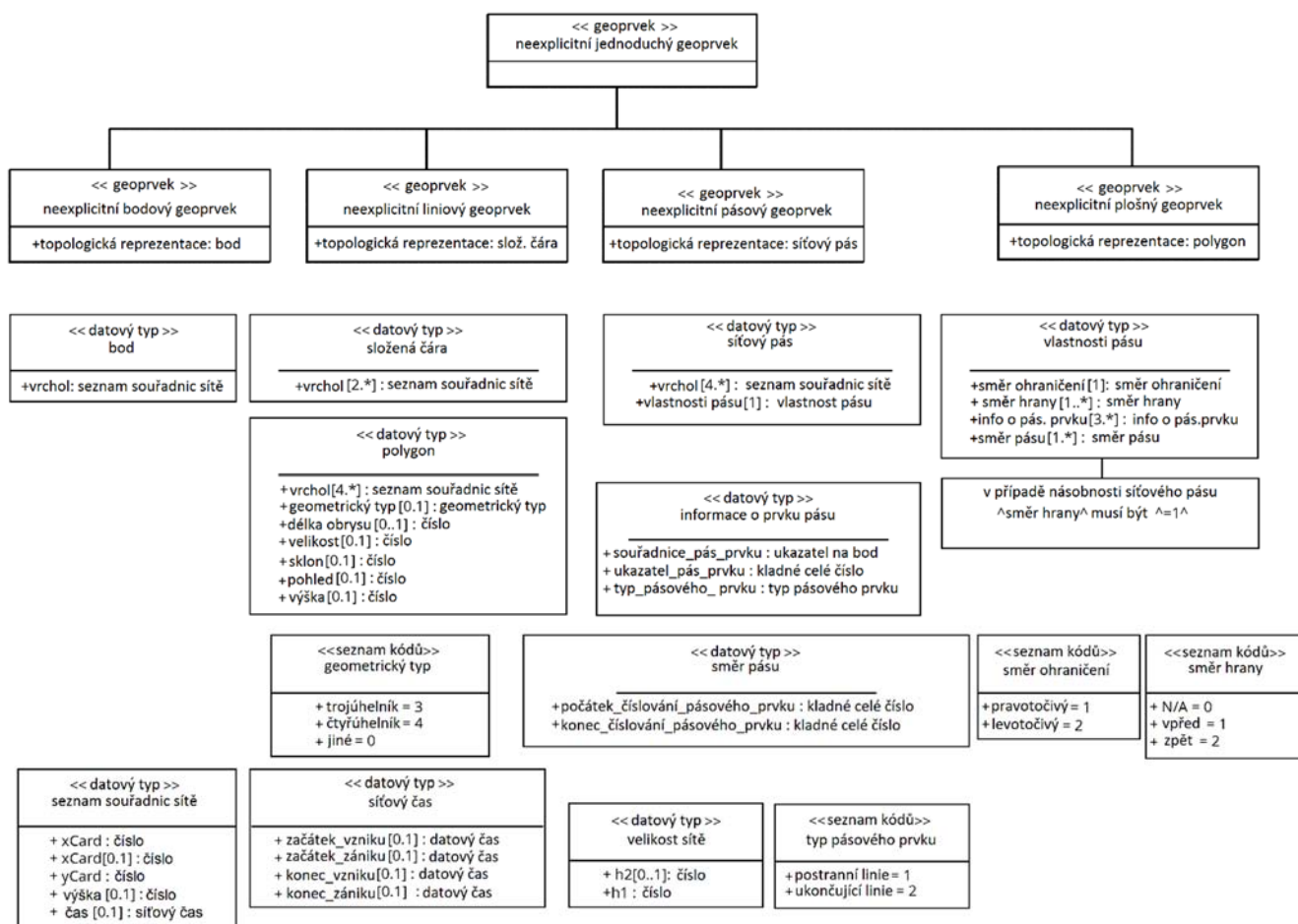
Obr. 3 - Konceptuální datový model jednoduchých geoprvků, ne-explicitní topologie
